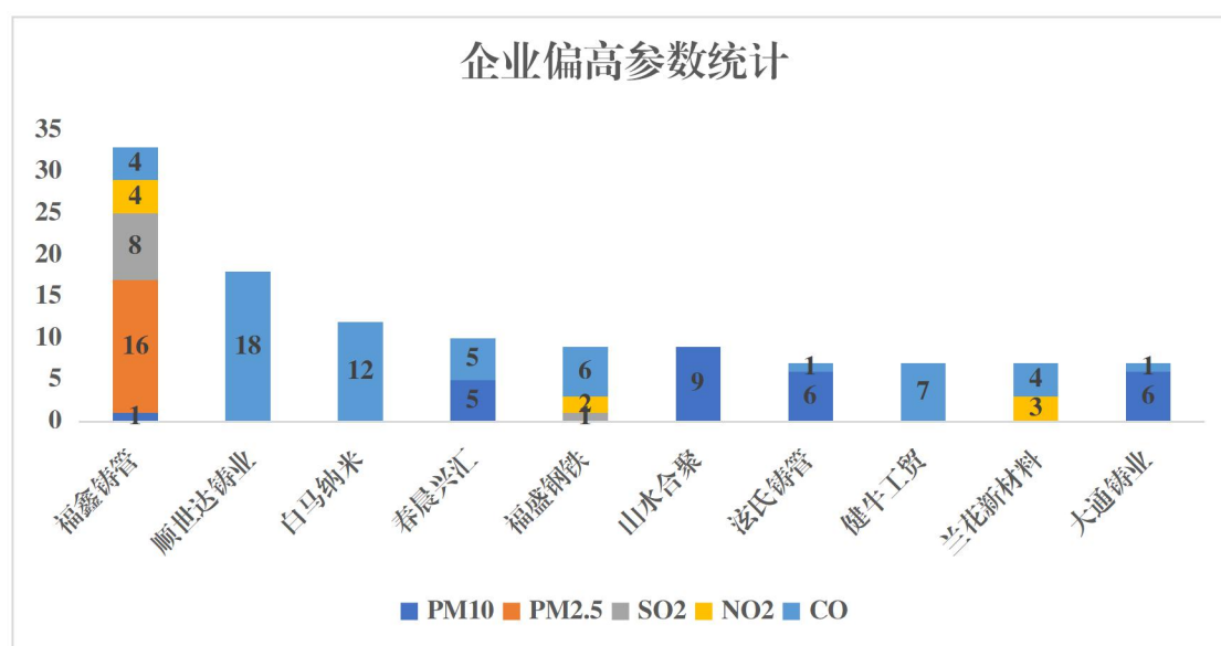
图2 2020年8月晋城市重点涉气企业污染参数异常情况
