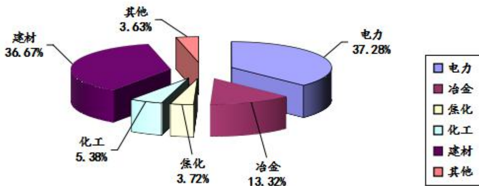
图2：2026年第2季度晋城市监控企业废气氮氧化物排放量各行业占比图
