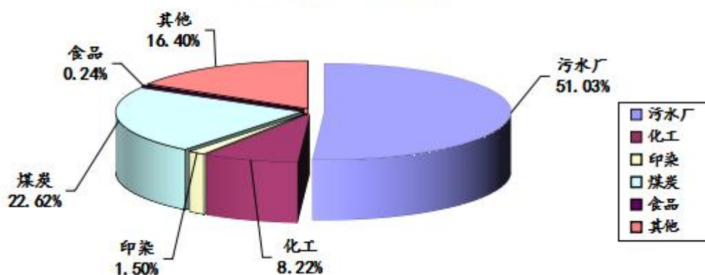
图5:2026年第2季度晋城市监控企业废水氨氮 排放量各行业占比图
