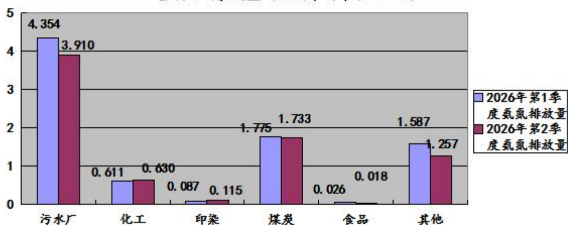
图26: 2026年第2季度晋城市监控企业废水氨氮 各行业排放量环比图 (单位: 吨)
