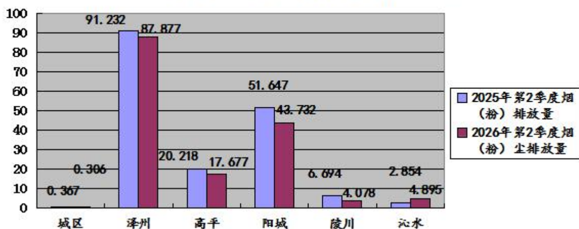
图21:2026年第2季度晋城市各县（市、区）监控企业废气烟（粉）尘排放量同比图（单位：吨）
