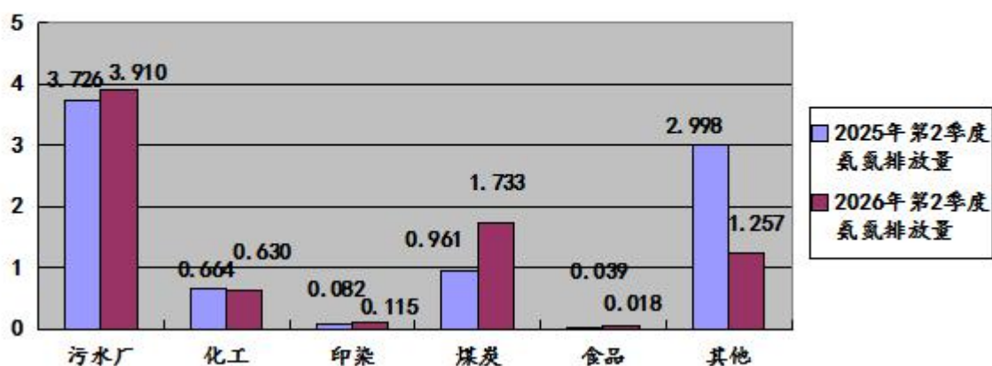
图25:2026年第2季度晋城市监控企业废水氨氮 各行业排放量同比图 (单位: 吨)
