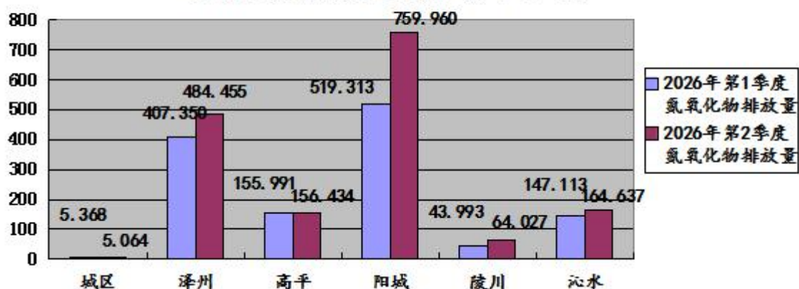
图20:2026年第2季度晋城市各县（市、区）监控企业废气氮氧化物排放量环比图（单位：吨）
