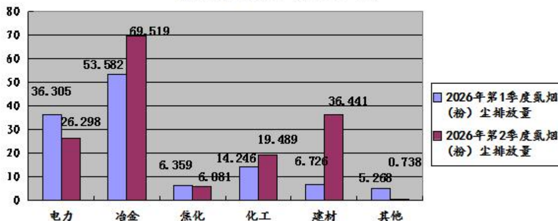
图13: 2026年第2季度晋城市监控企业废气烟(粉)尘排放量环比图 (单位: 吨)
