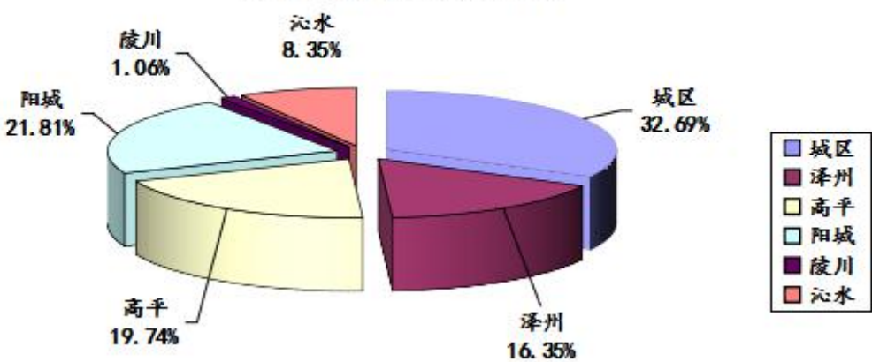
图28: 2026年第2季度晋城市各县（市、区）监控企业 废水氨氮排放量占比图
