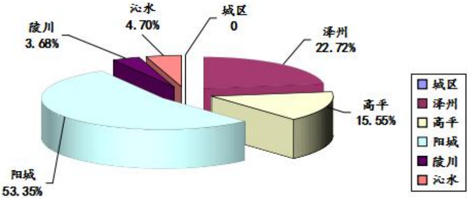
图14:2026年第2季度晋城市各县（市、区）监控企业废气 二氧化硫排放量占比图
