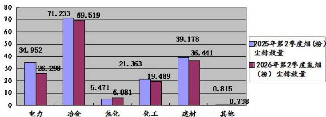
图12: 2026年第2季度晋城市监控企业废气烟(粉)尘排放量同比图 (单位: 吨)
