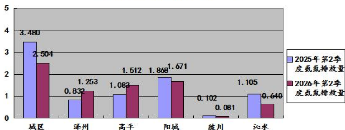
图31：2026年第2季度晋城市各县(市、区)监控企业废水 氨氮排放量同比图（单位：吨）
