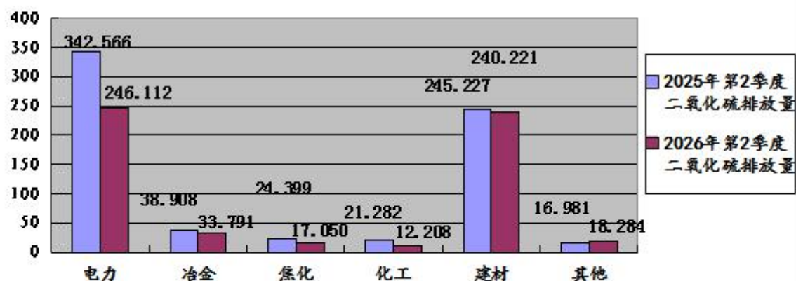
图8:2026年第2季度晋城市监控企业废气二氧化硫 排放量同比图 (单位:吨)
