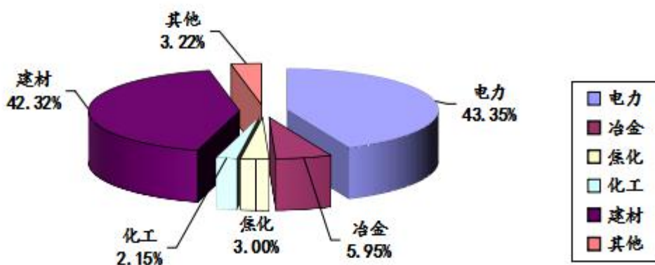
图1：2026年第2季度晋城市监控企业废气二氧化硫排放量各行业占比图
