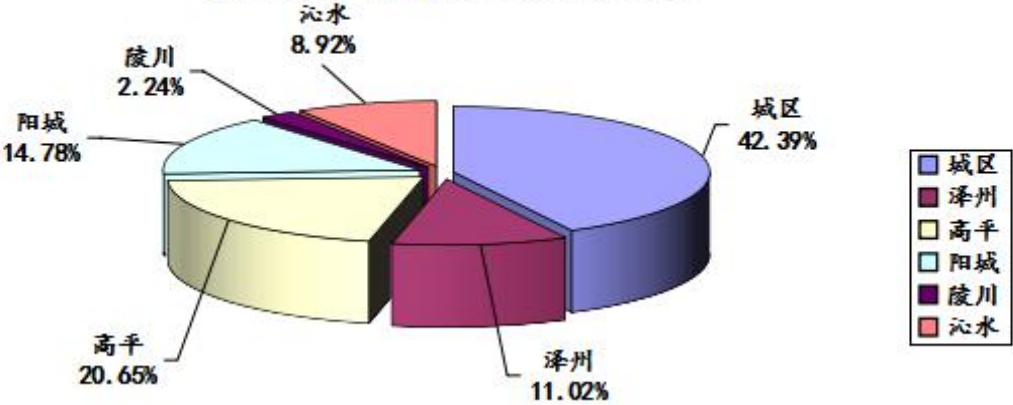
图27:2026年第2季度晋城市各县（市、区）监控企业 废水化学需氧量排放量占比图
