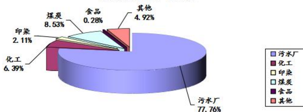
图4:2026年第2季度晋城市监控企业废水化学需氧量 排放量各行业占比图
