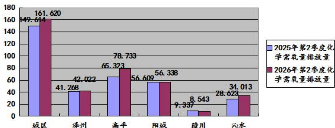
图29：2026年第2季度晋城市各县(市、区)监控企业废水 化学需氧量排放量同比图（单位：吨）
