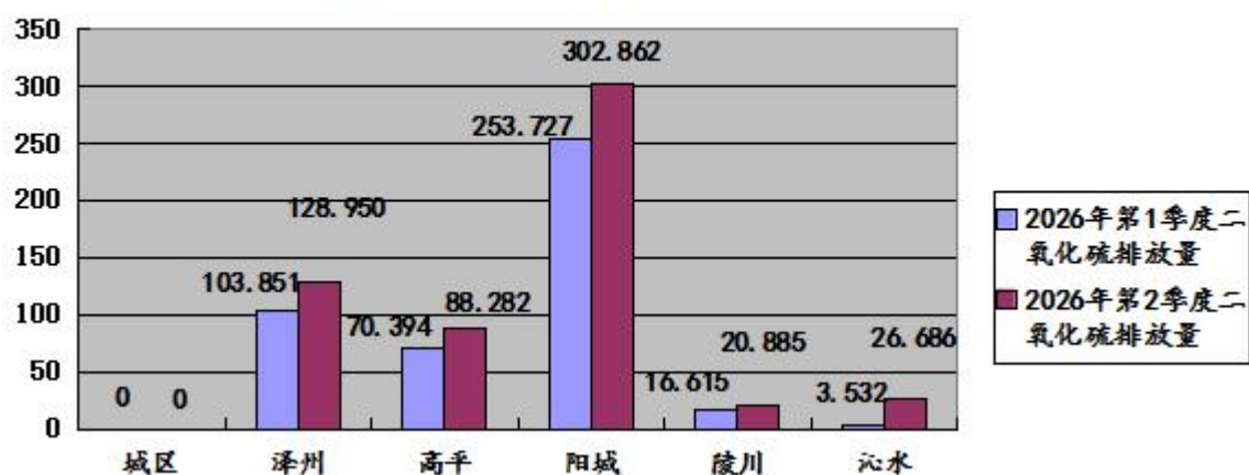
图18:2026年第2季度晋城市各县（市、区）监控企业废气二氧化硫排放量环比图（单位：吨）
