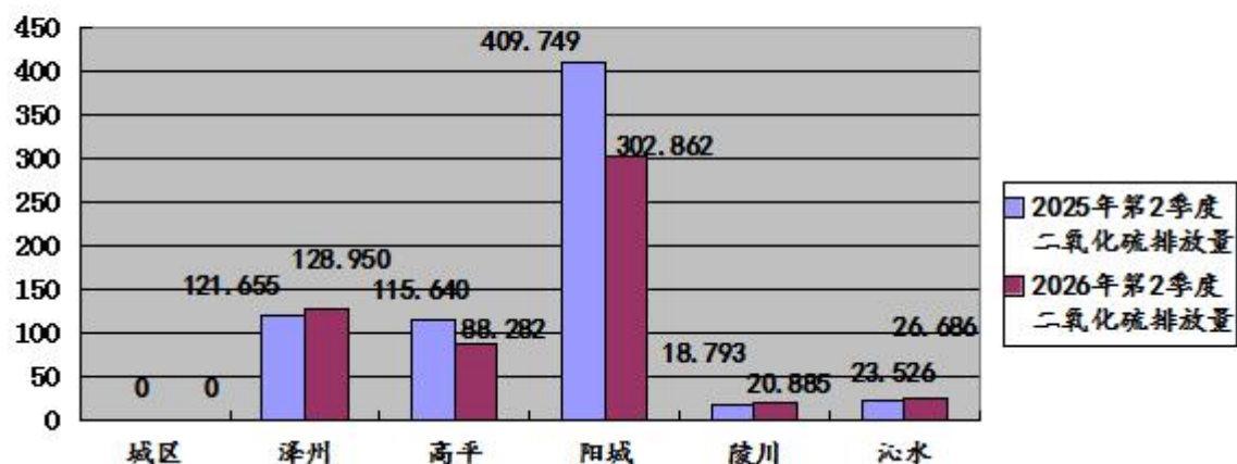
图17:2026年第2季度晋城市各县（市、区）监控企业废气二氧化硫排放量同比图（单位：吨）
