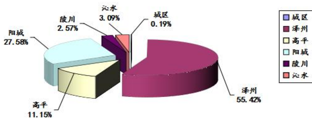
图16:2026年第2季度晋城市各县（市、区）监控企业废气烟（粉）尘排放量占比图
