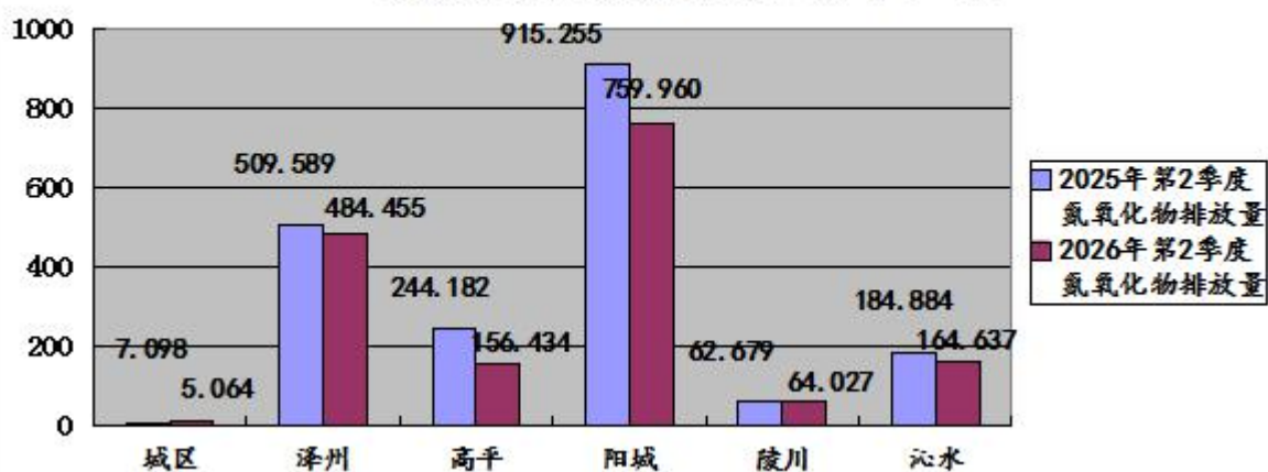
图19:2026年第2季度晋城市各县（市、区）监控企业废气氮氧化物排放量同比图（单位：吨）
