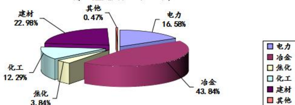
图3：2026年第2季度晋城市监控企业烟（粉）尘排放量各行业占比图
