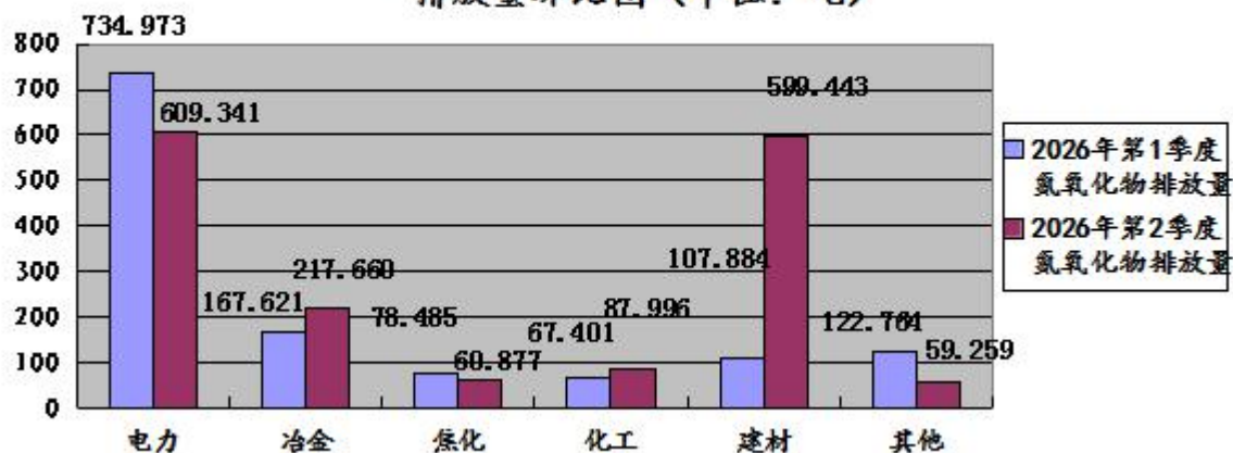
图11: 2026年第2季度晋城市监控企业废气氮氧化物排放量环比图 (单位: 吨)
