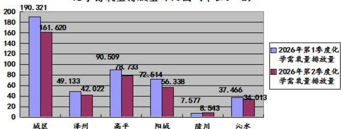
图30：2026年第2季度晋城市各县(市、区)监控企业废水 化学需氧量排放量环比图（单位：吨）
