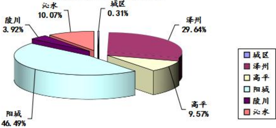
图15:2026年第2季度晋城市各县（市、区）监控企业废气 氮氧化物排放量占比图
