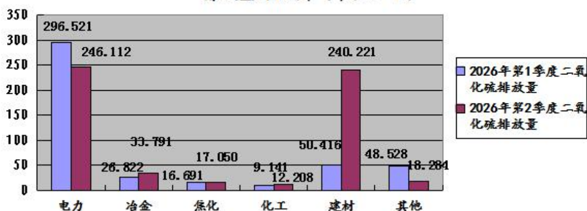
图9: 2026年第2季度晋城市监控企业废气二氧化硫 排放量环比图 (单位:吨)
