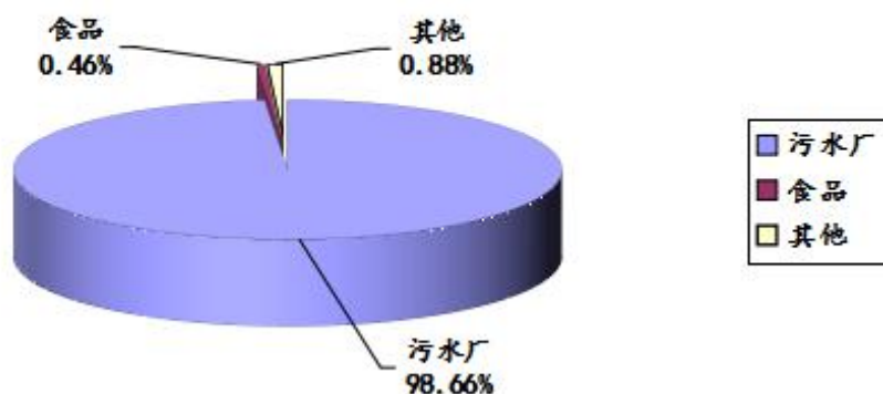
图6:2026年第2季度晋城市监控企业废水总磷 排放量各行业占比图
