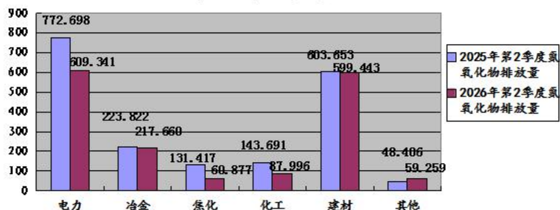
图10:2026年第2季度晋城市监控企业废气氮氧化物 排放量同比图 (单位:吨)
