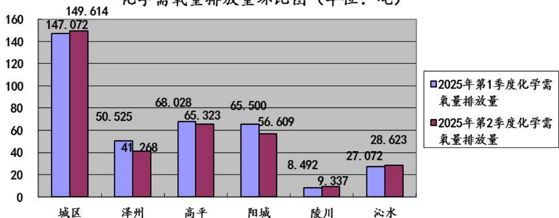
图30：2025年第2季度晋城市各县(市、区)监控企业废水 化学需氧量排放量环比图（单位：吨）
