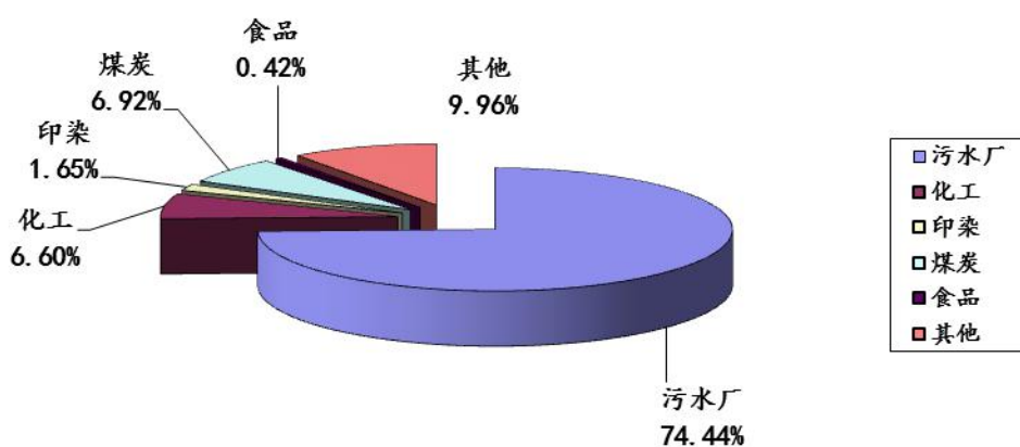
图4:2025年第2季度晋城市监控企业废水化学需氧量排放量各行业比较图
