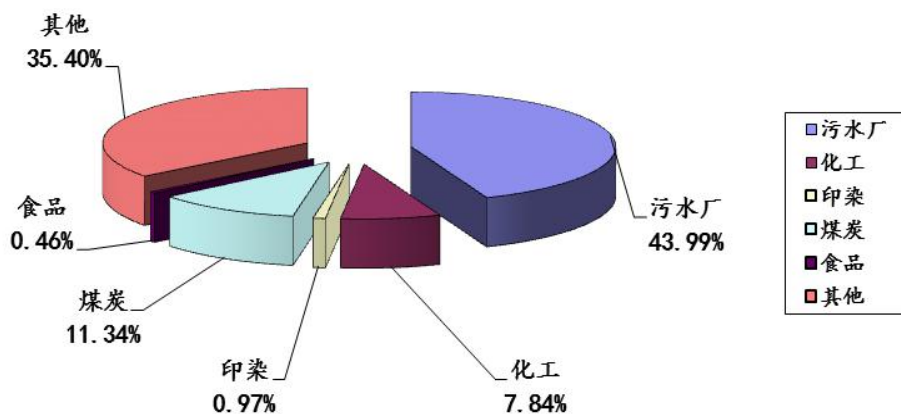
图5:2025年第2季度晋城市监控企业废水氨氮排放量各行业比较图
