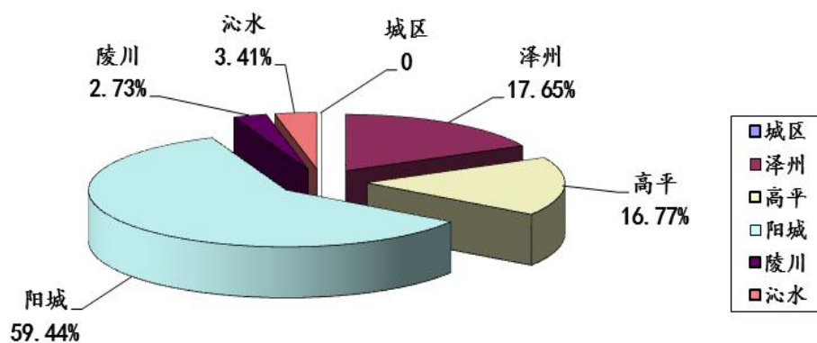
图14:2025年第2季度晋城市各县（市、区）监控企业废气 二氧化硫排放量占比图
