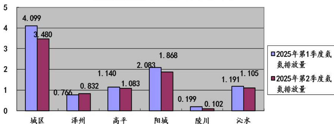
图32：2025年第2季度晋城市各县(市、区)监控企业废水 氨氮排放量环比图（单位：吨）
