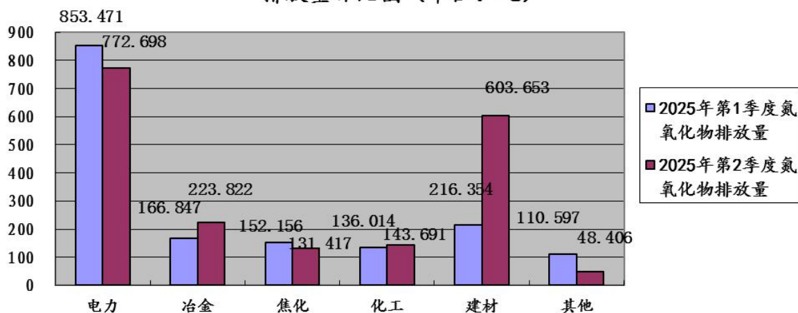
图11: 2025年第2季度晋城市监控企业废气氮氧化物 排放量环比图 (单位:吨)
