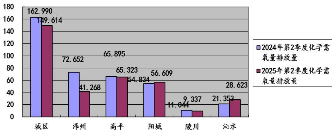
图29: 2025年第2季度晋城市各县(市、区)监控企业废水 化学需氧量排放量同比图（单位：吨）
