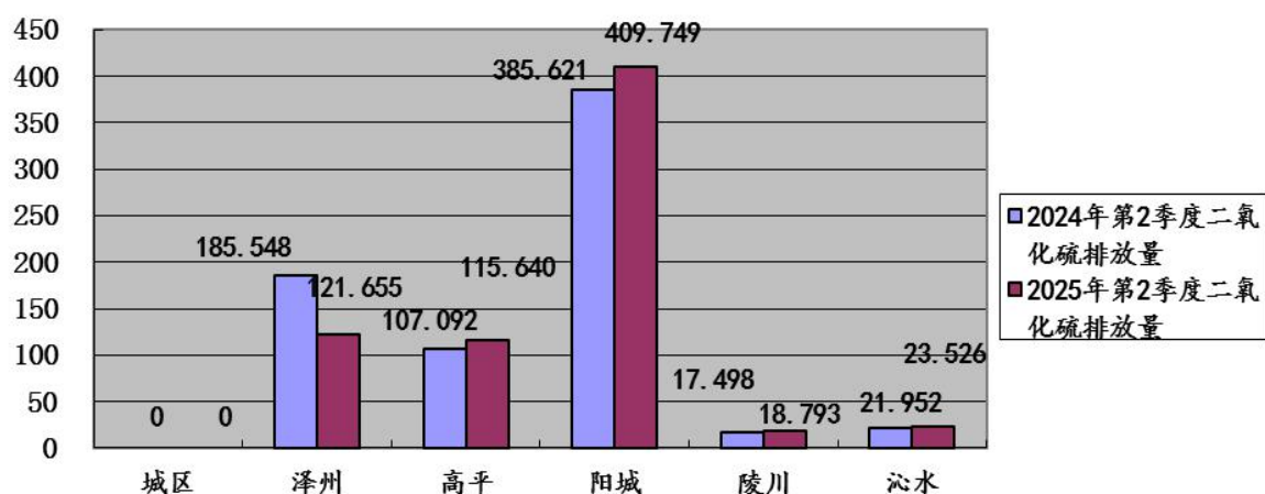
图17:2025年第2季度晋城市各县（市、区）监控企业废气 二氧化硫排放量同比图（单位：吨）
