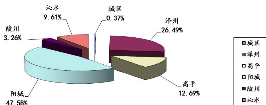
图15:2025年第2季度晋城市各县（市、区）监控企业废气 氮氧化物排放量占比图
