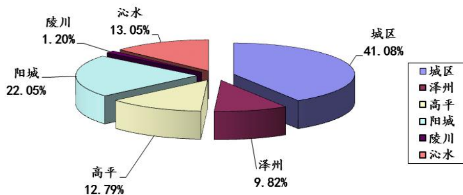
图28: 2025年第2季度晋城市各县（市、区）监控企业 废水氨氮排放量比较图
