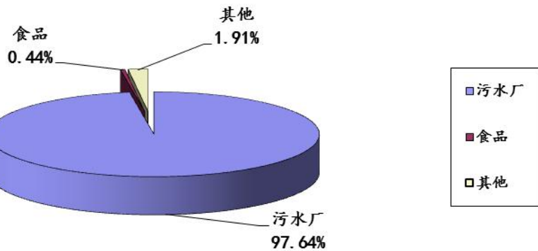
图7:2025年第2季度晋城市监控企业废水总氮 排放量各行业比较图
