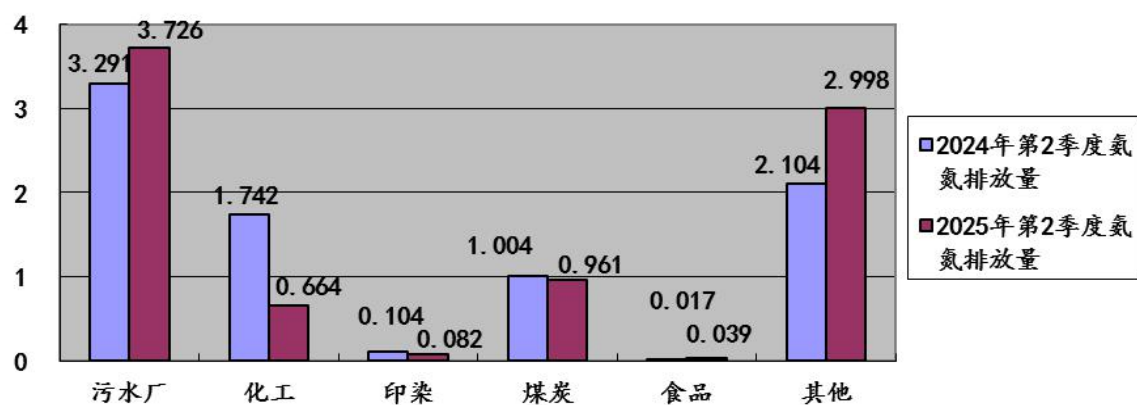
图25:2025年第2季度晋城市监控企业废水氨氮 各行业排放量同比图（单位：吨）
