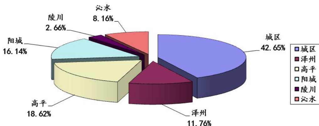
图27:2025年第2季度晋城市各县（市、区）监控企业 废水化学需氧量排放量比较图
