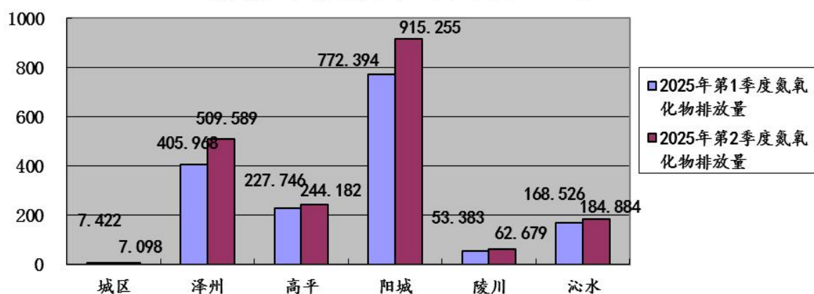
图20:2025年第2季度晋城市各县（市、区）监控企业废气 氮氧化物排放量环比图（单位：吨）
