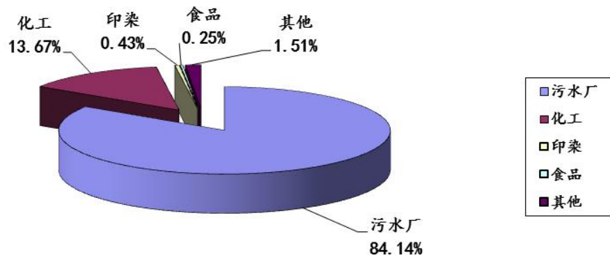
图7:2025年第2季度晋城市监控企业废水总氮 排放量各行业比较图
