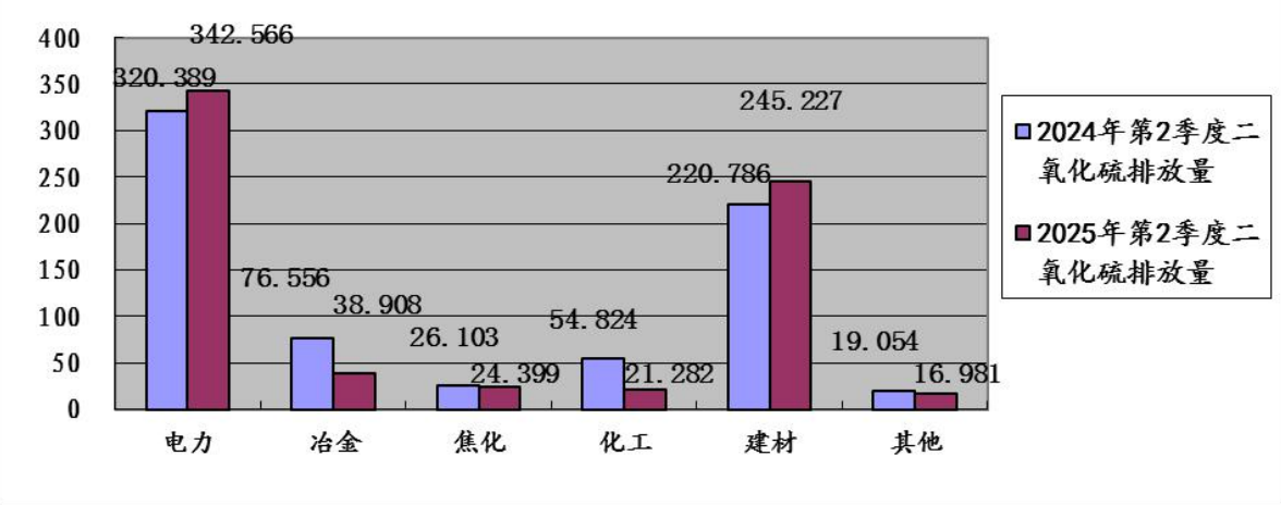
图8:2025年第2季度晋城市监控企业废气二氧化硫排放量同比图（单位：吨）
