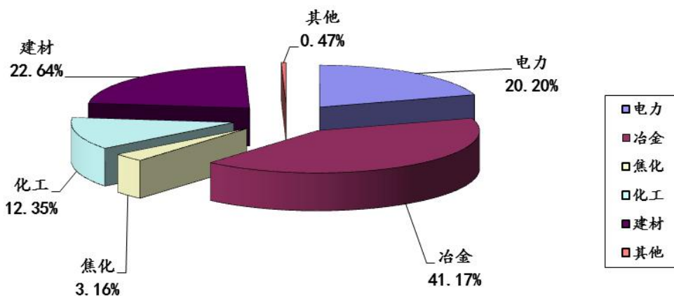
图3：2025年第2季度晋城市监控企业烟（粉）尘排放量各行业占比图
