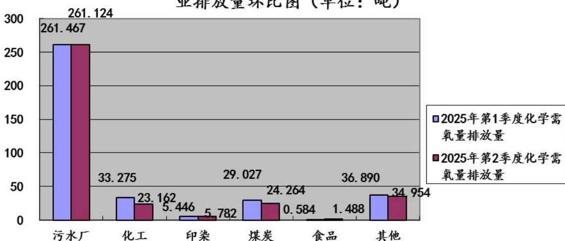
图24: 2025年第2季度晋城市监控企业废水化学需氧量各行 业排放量环比图（单位：吨）
