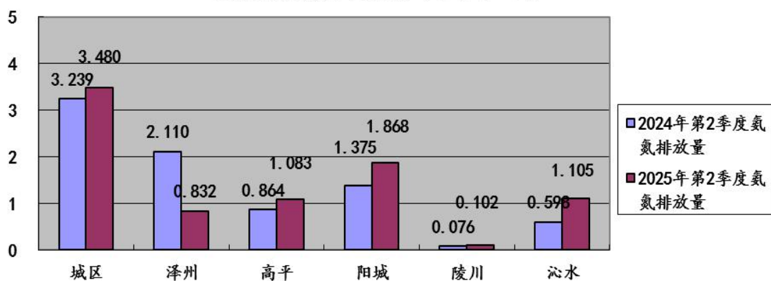
图31：2025年第2季度晋城市各县(市、区)监控企业废水 氨氮排放量同比图（单位：吨）
