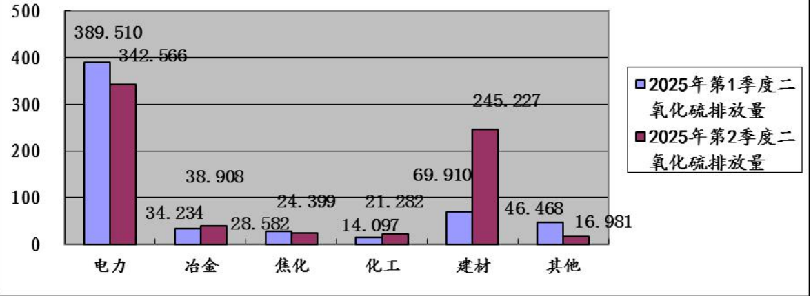
图9：2025年第2季度晋城市监控企业废气二氧化硫排放量环比图（单位：吨）
