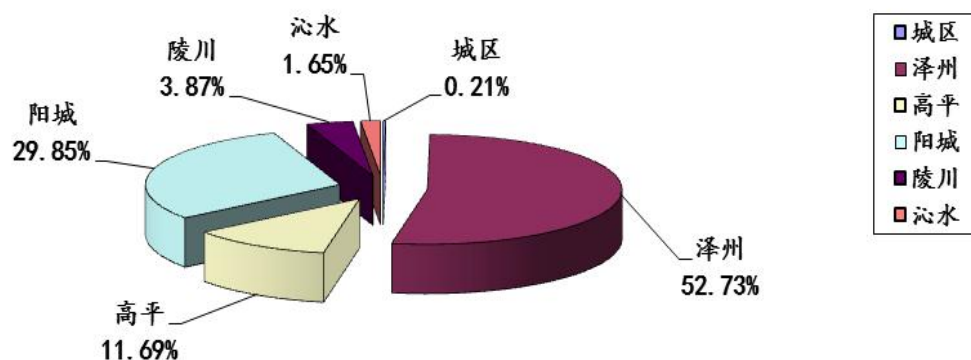
图16:2025年第2季度晋城市各县（市、区）监控企业废气 烟（粉）尘排放量占比图
