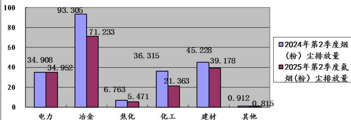
图12:2025年第2季度晋城市监控企业废气烟(粉)尘 排放量同比图 (单位:吨)
