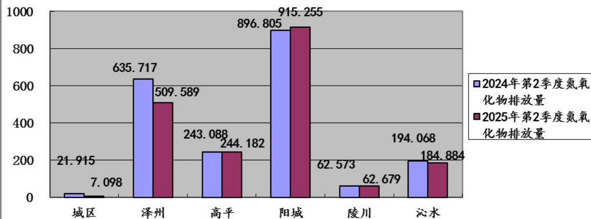
图19:2025年第2季度晋城市各县（市、区）监控企业废气 氮氧化物排放量同比图（单位：吨）
