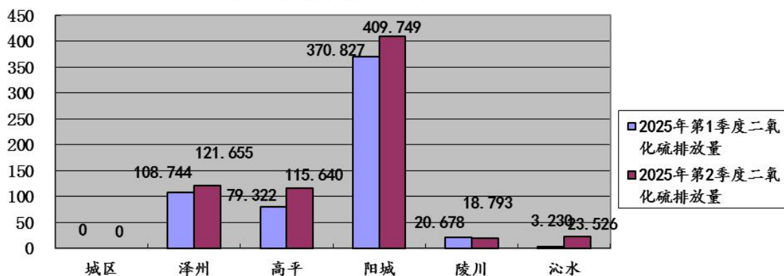
图18:2025年第2季度晋城市各县（市、区）监控企业废气 二氧化硫排放量环比图（单位：吨）
