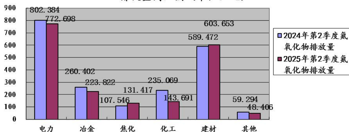
图10:2025年第2季度晋城市监控企业废气氮氧化物 排放量同比图 (单位:吨)
