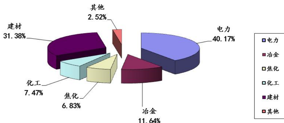
图2：2025年第2季度晋城市监控企业废气氮氧化物排放量各行业占比图
