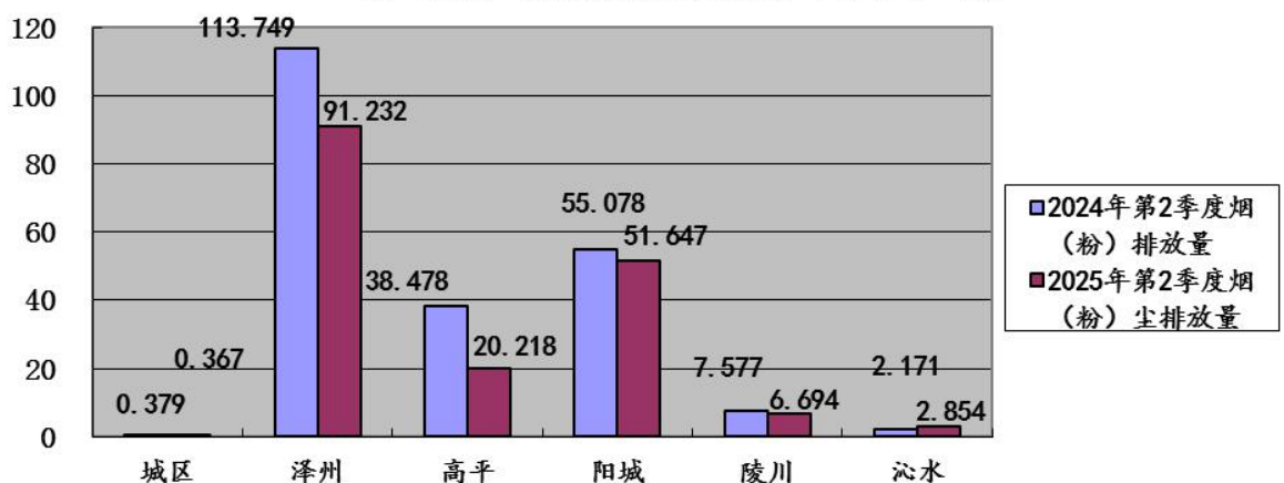
图21:2025年第2季度晋城市各县（市、区）监控企业废气 烟（粉）尘排放量同比图（单位：吨）
