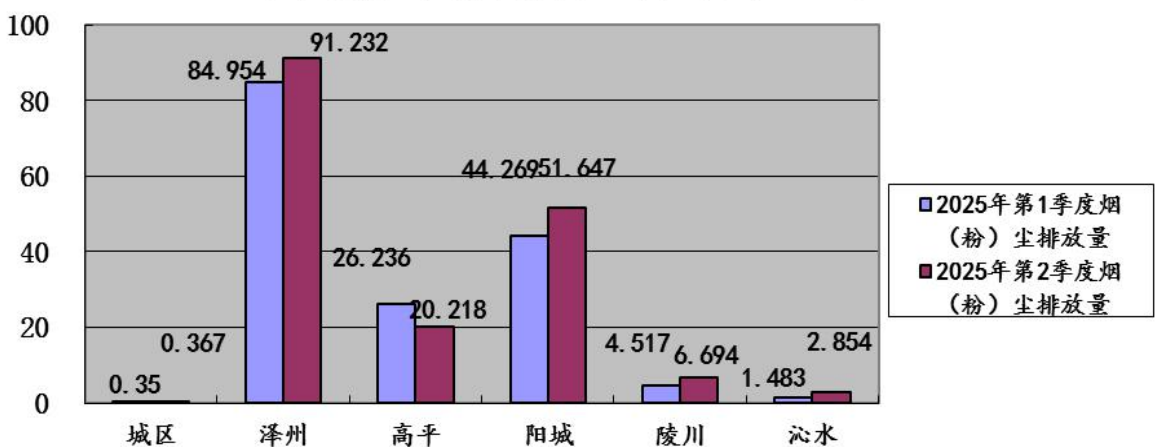
图22:2025年第2季度晋城市各县（市、区）监控企业废气 烟（粉）尘排放量环比图（单位：吨）
