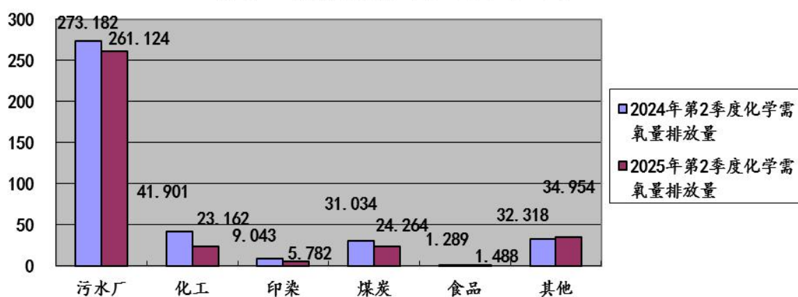
图23:2025年第2季度晋城市监控企业废水化学需氧量 各行业排放量同比图（单位：吨）
