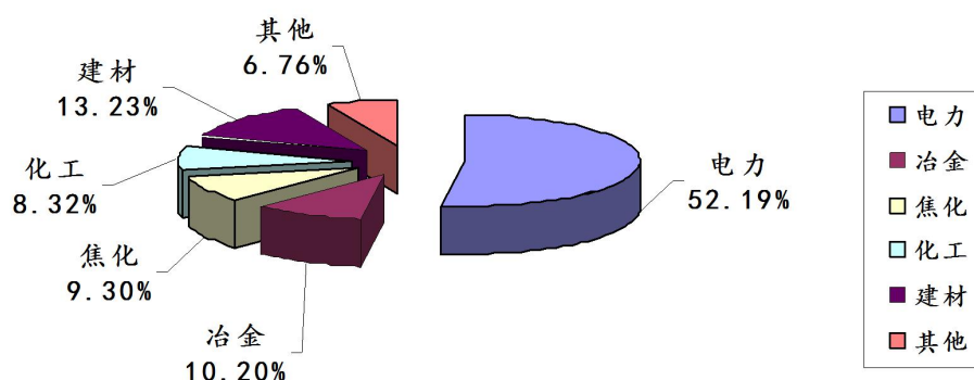
图2：2025年第1季度晋城市监控企业废气氮氧化物排放量各行业占比图
