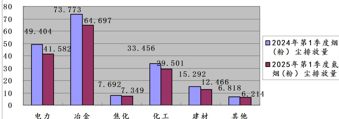
图12:2025年第1季度晋城市监控企业废气烟（粉）尘 排放量同比图（单位：吨）
