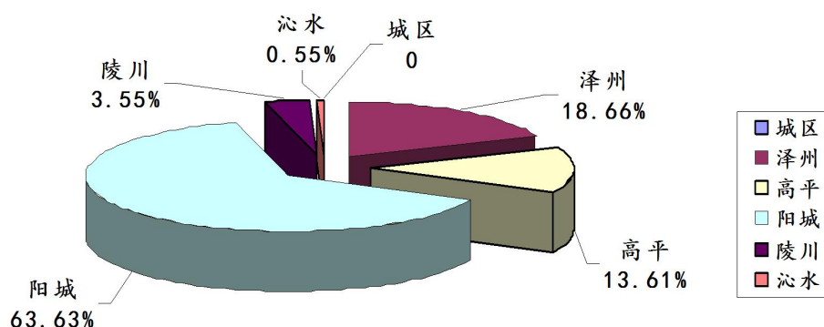
图14:2025年第1季度晋城市各县（市、区）监控企业废气二氧化硫排放量占比图
