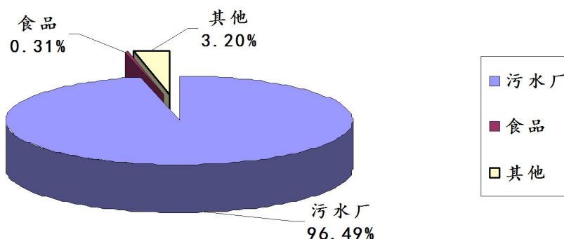
图7:2025年第1季度晋城市监控企业废水总氮排放量各行业比较图
