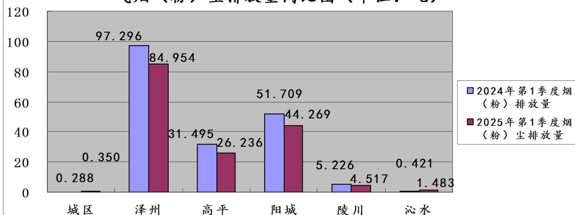
图21:2025年第1季度晋城市各县（市、区）监控企业废 气烟（粉）尘排放量同比图（单位：吨）
