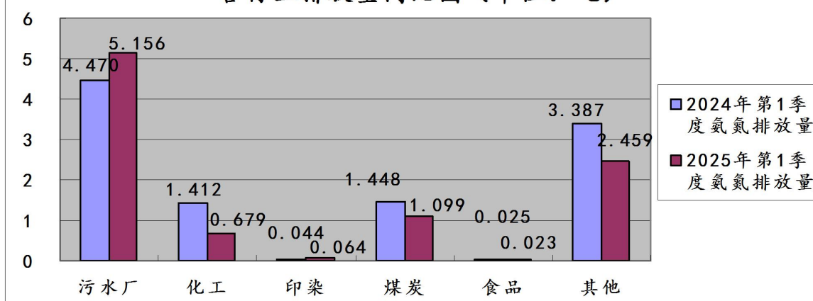
图25:2025年第1季度晋城市监控企业废水氨氮 各行业排放量同比图（单位：吨）
