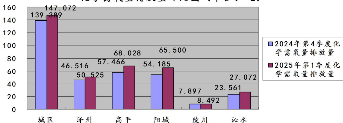
图30：2025年第1季度晋城市各县(市、区)监控企业废水 化学需氧量排放量环比图（单位：吨）
