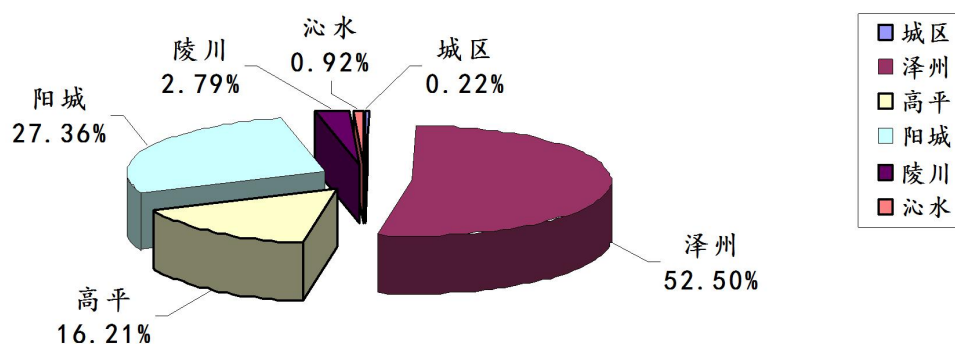
图16:2025年第1季度晋城市各县（市、区）监控企业废气烟（粉）尘排放量占比图
