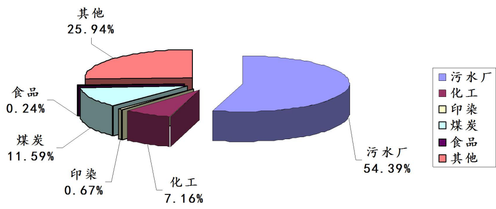
图5:2025年第1季度晋城市监控企业废水氨氮 排放量各行业比较图
