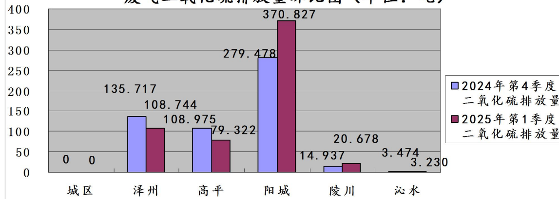
图18:2025年第1季度晋城市各县（市、区）监控企业废气二氧化硫排放量环比图（单位：吨）
