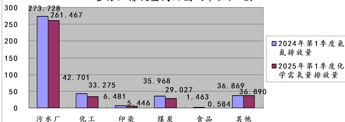
图23:2025年第1季度晋城市监控企业废水化学需氧量 各行业排放量同比图（单位：吨）
