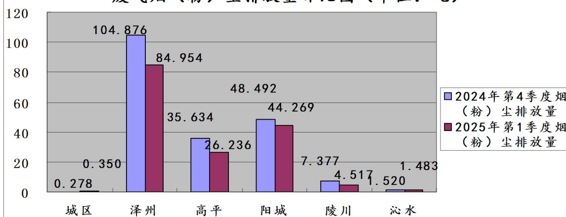
图22:2025年第1季度晋城市各县（市、区）监控企业 废气烟（粉）尘排放量环比图（单位：吨）
