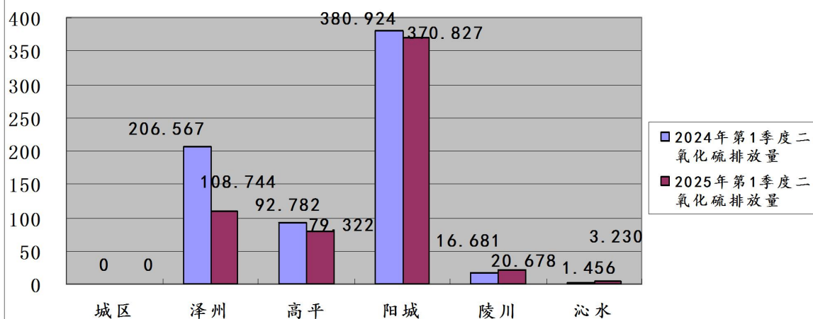
图17:2025年第1季度晋城市各县（市、区）监控企业废气二氧化硫排放量同比图（单位：吨）
