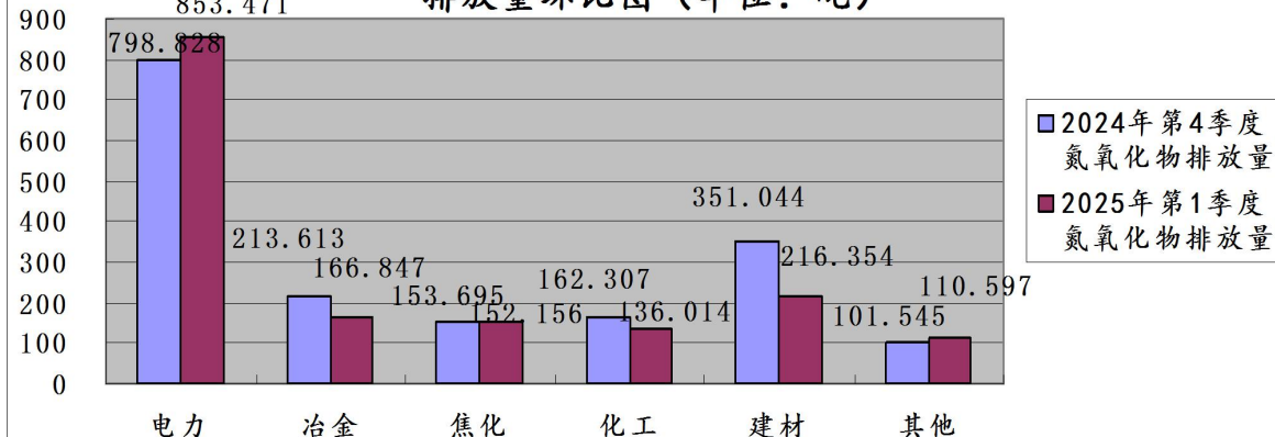
图11: 2025年第1季度晋城市监控企业废气氮氧化物 排放量环比图（单位：吨）
