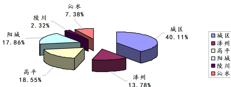
图27:2025年第1季度晋城市各县（市、区）监控企业 废水化学需氧量排放量比较图
