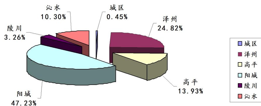
图15:2025年第1季度晋城市各县（市、区）监控企业废气氮氧化物排放量占比图
