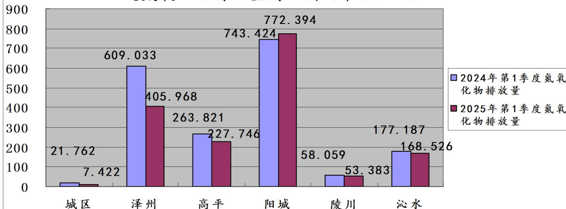
图19:2025年第1季度晋城市各县（市、区）监控企业废气氮氧化物排放量同比图（单位：吨）
