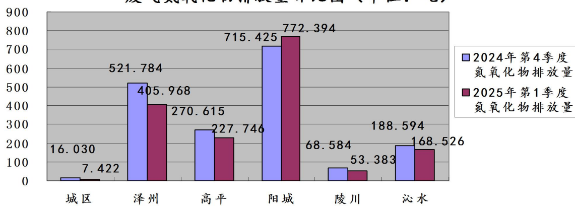
图20:2025年第1季度晋城市各县（市、区）监控企业 废气氮氧化物排放量环比图（单位：吨）
