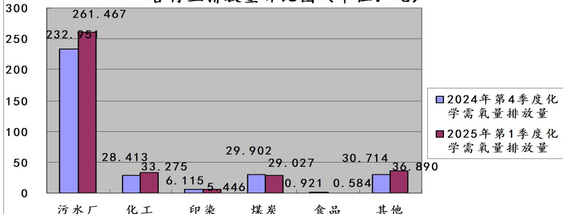
图24: 2025年第1季度晋城市监控企业废水化学需氧量 各行业排放量环比图（单位：吨）
