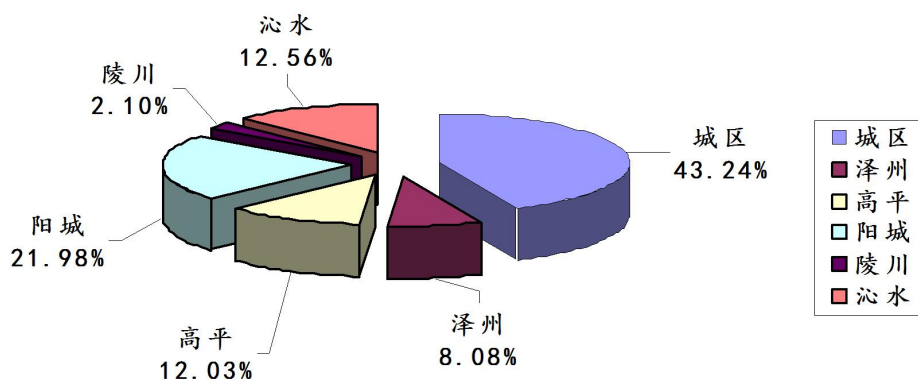
图28: 2025年第1季度晋城市各县（市、区）监控企业 废水氨氮排放量比较图
