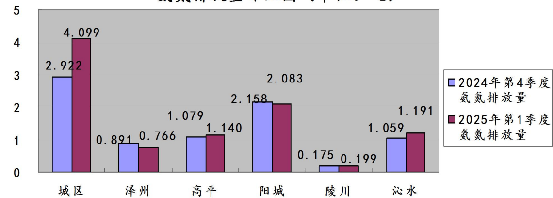
图32：2025年第1季度晋城市各县(市、区)监控企业废水 氨氮排放量环比图（单位：吨）
