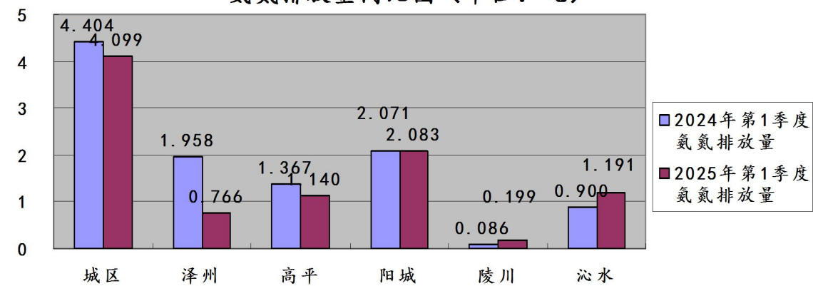
图31：2025年第1季度晋城市各县(市、区)监控企业废水 氨氮排放量同比图（单位：吨）
