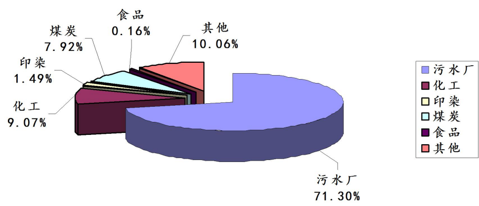
图4:2025年第1季度晋城市监控企业废水化学需氧量 排放量各行业比较图
