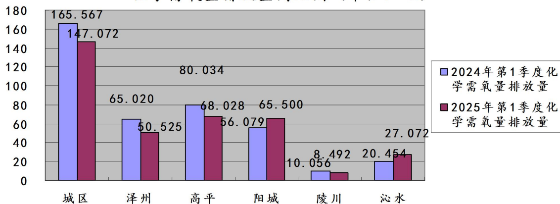
图29: 2025年第1季度晋城市各县(市、区)监控企业废水 化学需氧量排放量同比图 (单位: 吨)
