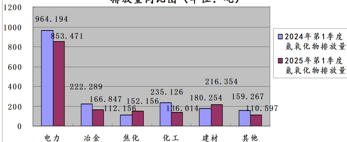
图10:2025年第1季度晋城市监控企业废气氮氧化物 排放量同比图（单位：吨）
