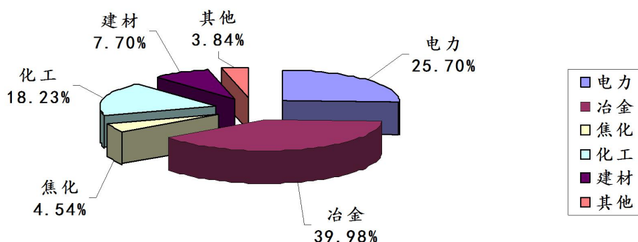
图3：2025年第1季度晋城市监控企业烟（粉）尘排放量各行业占比图
