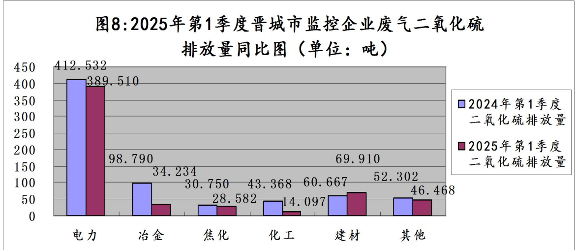
图9: 2025年第1季度晋城市监控企业废气二氧化硫排放量环比图（单位：吨）
